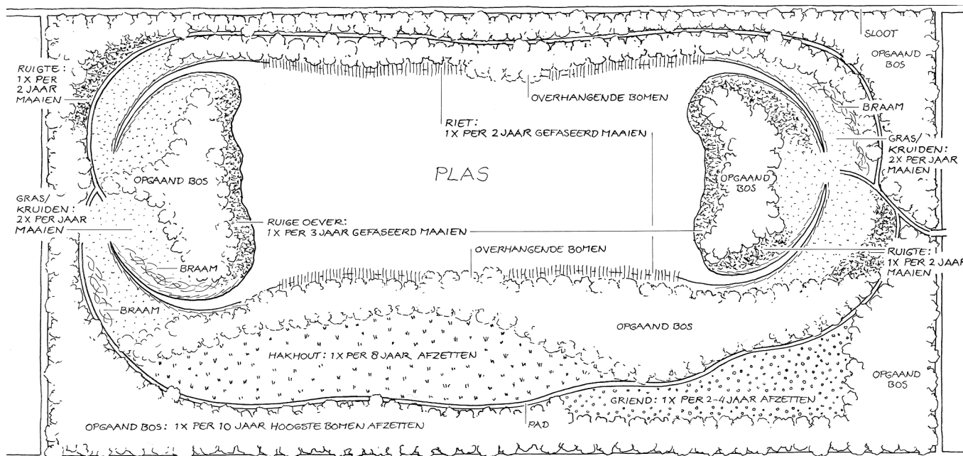
Voorbeeld van een eendekooi, roggenei-model
